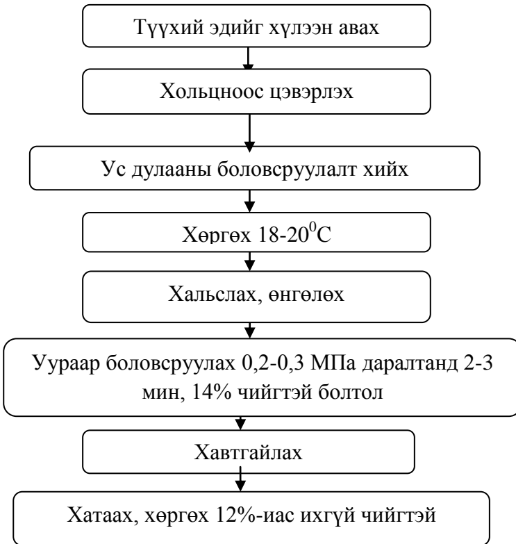
Зураг 1. Хошуу тарианы хавтгайлсан бэлдмэл үйлдвэрлэх технологийн бүдүүвч
